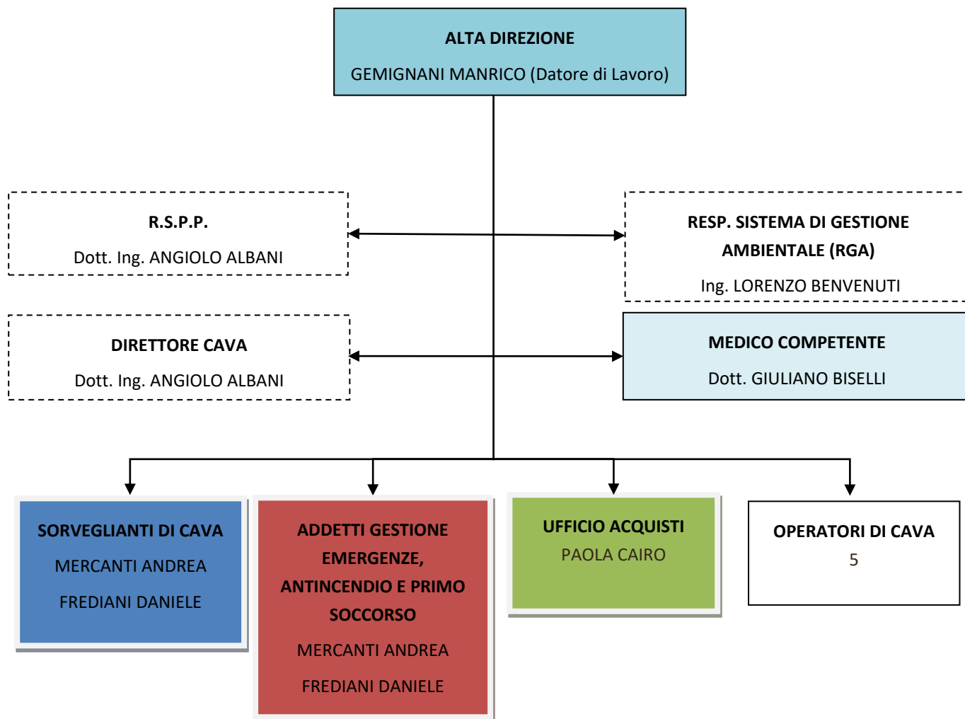
Fig. 7 - Organigramma
